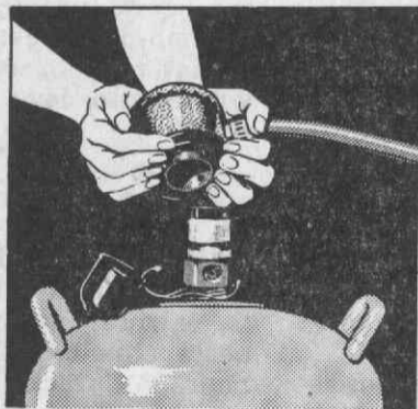
1 — O regulador é aplicado na válvula com o anel preto de plástico levantado.
