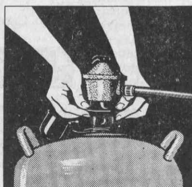
3 — Carregando no anel preto até se ouvir um «click», o regulador fica pronto a funcionar.
