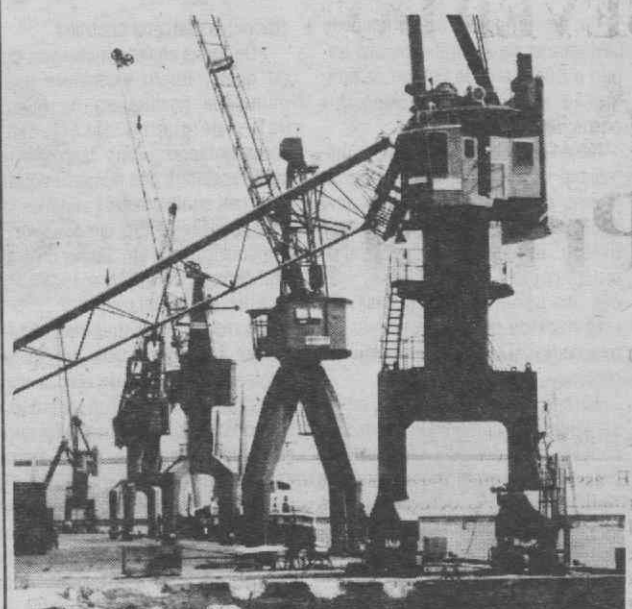
No cais comercial dois novos guindastes electricos estão a ser montados (na foto localizam-se nos extremos) com possibilidade de movimentar carga ate 12 toneladas num espaço de 16 metros. Este moderno equipamento dara ao porto da Figueira da Foz uma capacidade de resposta significativa, especialmente no tipo de produtos que são escoados por este porto.
