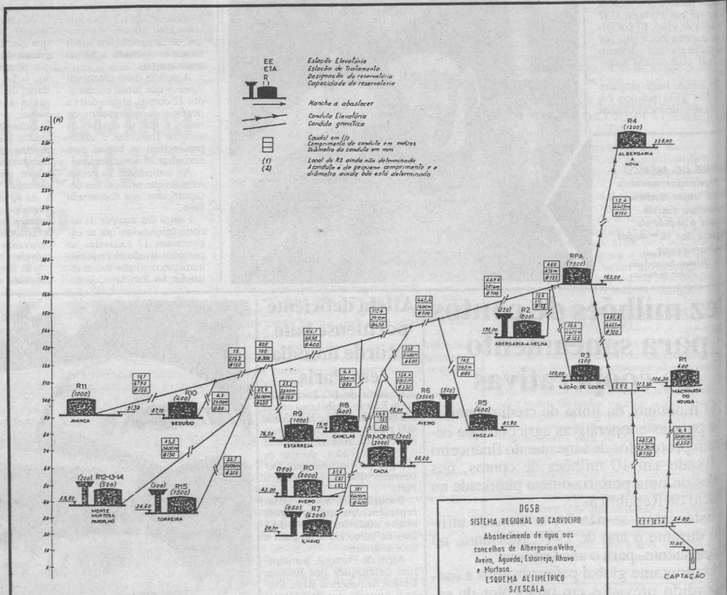
O plano do Sistema Regional do Carvoeiro. A solução para o abastecimento de água a uma vasta franja populacional da região de Aveiro
