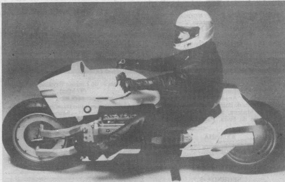
Uma nova concepção de motocicleta com propulsão BMW K 100. Um estudo de forma como tese de diplomação, da República Federal da Alemanha.
