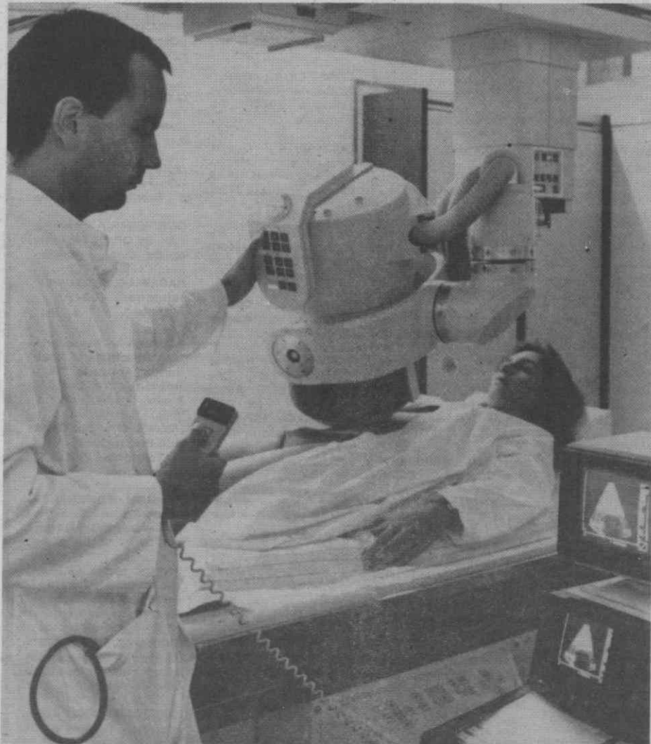
A foto dá um exemplo de aproveitamento médico da técnica para fins terapêuticos múltiplos. Esta aparelhagem permite a eliminação de cálculos nos rins e na vesícula biliar, e até no baço, por meio de ondas de choque. O médico pode optar entre raio X e ultrassom quando localiza o cálculo e controla o tratamento. Este novo aparelho combinado é o primeiro do mundo no género, combinando tipos diferentes de monitorização. Desta maneira, o médico, pode escolher o melhor modo de controlo segundo o caso a ser tratado. Em geral, os cálculos nos rins, nos canais biliares e no baço são detectados com o auxílio do raio X. Já na vesícula a posição exacta dos cálculos é determinada por meio de ultrassom. O médico guia-se pela imagem de ultrassom para controlar o emissor de ondas de choque.
