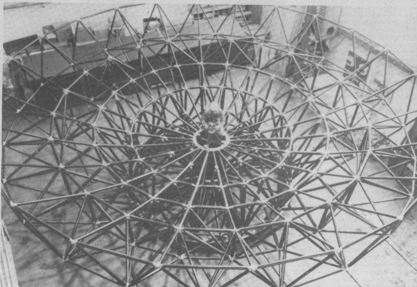
O radiotelescópio com estrutura de fibra sintética construído pela Krupp para ser instalado no alto de uma montanha no Arizona.
