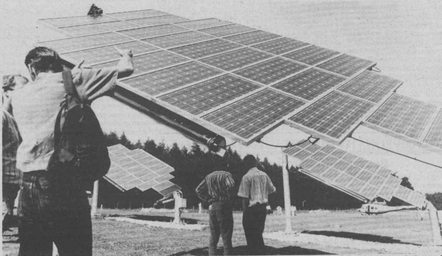
Colectores solares que se ajustam à posição do Sol com auxílio de sensores e sistemas hidráulicos (foto), produzindo assim 1/3 a mais de energia que instalações convencionais. Esta mais moderna fábrica solar da Europa encontra-se em Merklingen, no sul da Alemanha. Ela produz por ano 12.000 kw/h de electricidade. Para regiões de fraca infra-estrutura em países em desenvolvimento, a técnica solar pode significar uma importante ajuda.
